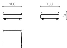
COD. N167011 pouf | pouf
